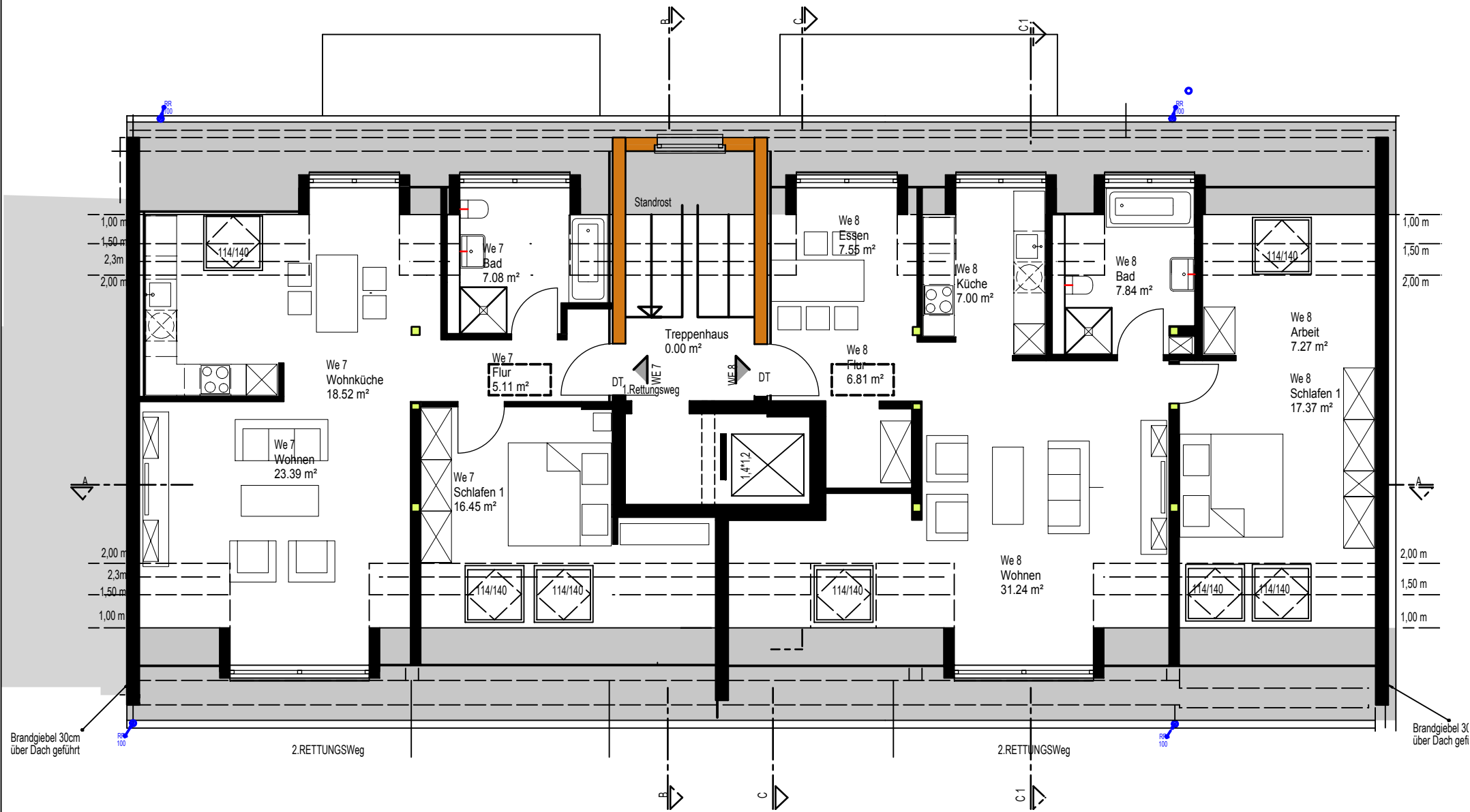
Dachgeschoss Wallstr. 10-12
